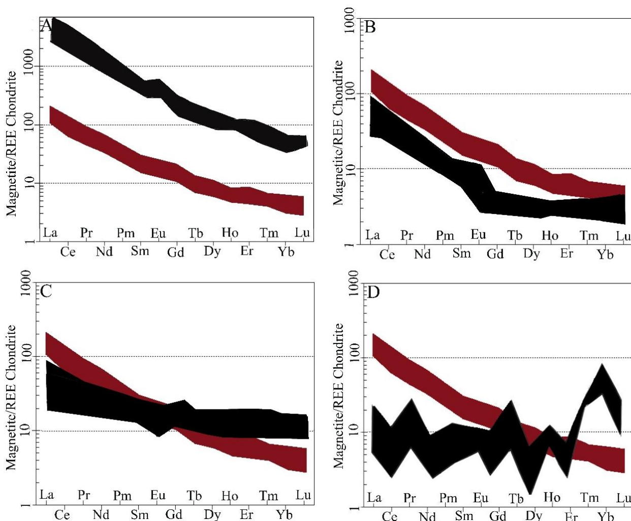
شکل ۱۴- مقایسه الگوی پراکندگی عنصرهای کمیاب بهنجارشده به ترکیب کندریت در منطقه نرم: (A) الگوی پراکندگی عنصرهای REE در کانسنگ مگنتیتی اندوخته‌های معدنی آهن گرمایی (Tallarico et al. , 2005); (B) الگوی پراکندگی عنصرهای REE در نمونه‌های کانسنگ آهن تیپ کایرونا (Frietsch and Pendahl, 1995); (C) الگوی پراکندگی REE در آهن اسکارنی می‌سی (Niiranen et al. , 2005); (D) الگوی پراکندگی REE در نمونه‌های مگنتیتی کانسارهای آهن رسوبی (Oksuz and Koc, 2009)
