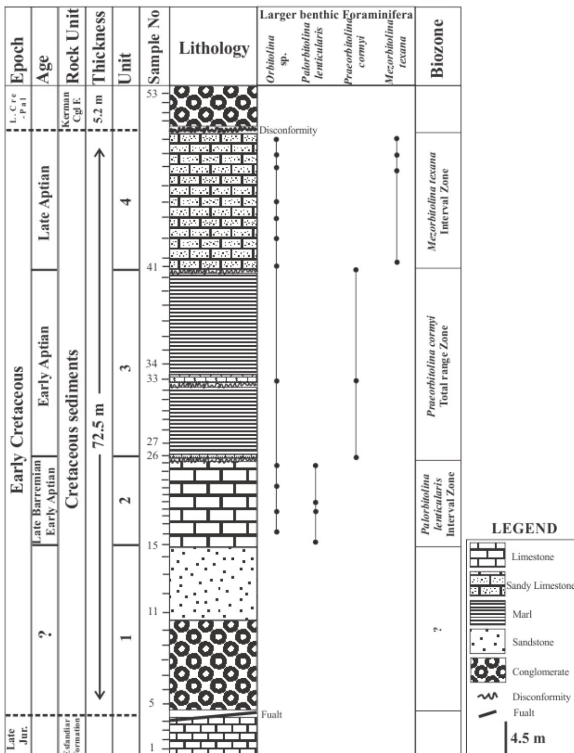
شکل ۳. ستون چینه سنگی و گسترش چینه‌نگاری گونه‌های اربیتولینید در نهشته‌های کرتاسه زیرین برش دیهوک
