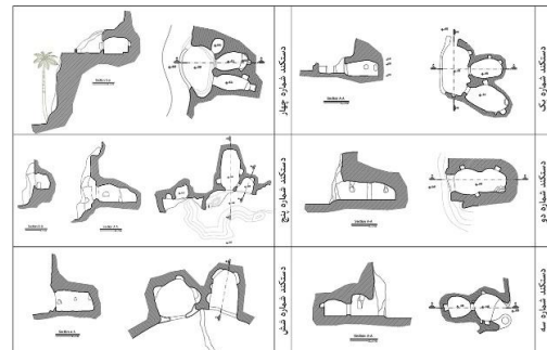
ت ۱۶. پلان و برش تعدادی از دستکندهای حاشیه جنوبی روستا. منبع: نگارندگان.
