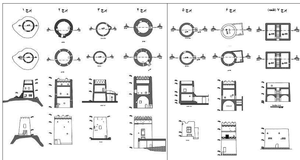
ت ۱۴. پلان و مقاطع برج‌های نگهبانی نابیند. منبع: نگارندگان.
