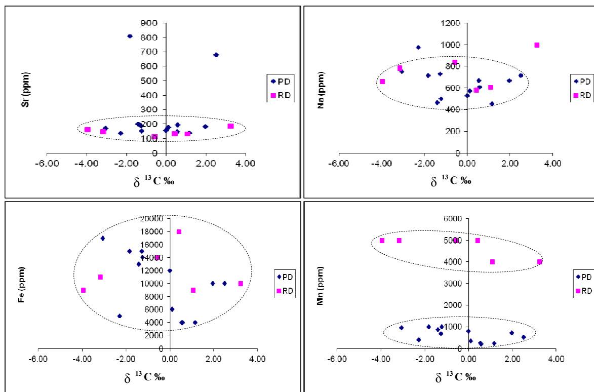
شکل ۷ نمودارهای پراکندگی عناصر استرانسیوم، سدیم، آهن و منگنز نسبت به \delta^{13}C در دولومیت‌های نوع PD و RD. در نمودارها نیز به استثنای منگنز، عناصر دیگر از محدوده‌ی مشترکی برخوردارند.
